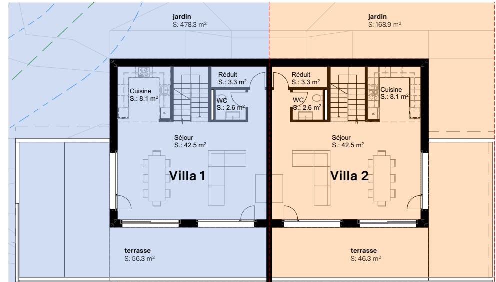
REZ SUPÉRIEUR
