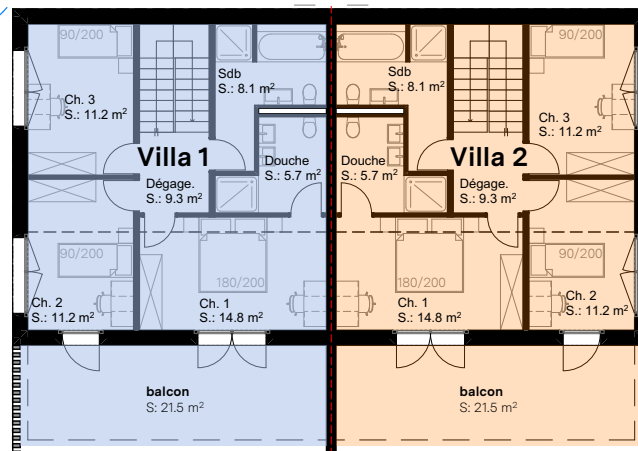
ÉTAGE
