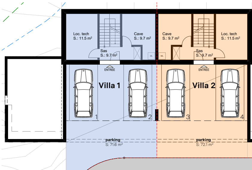
REZ INFÉRIEUR
